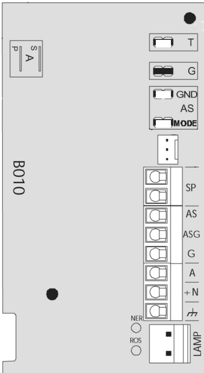
Bornier sirène
